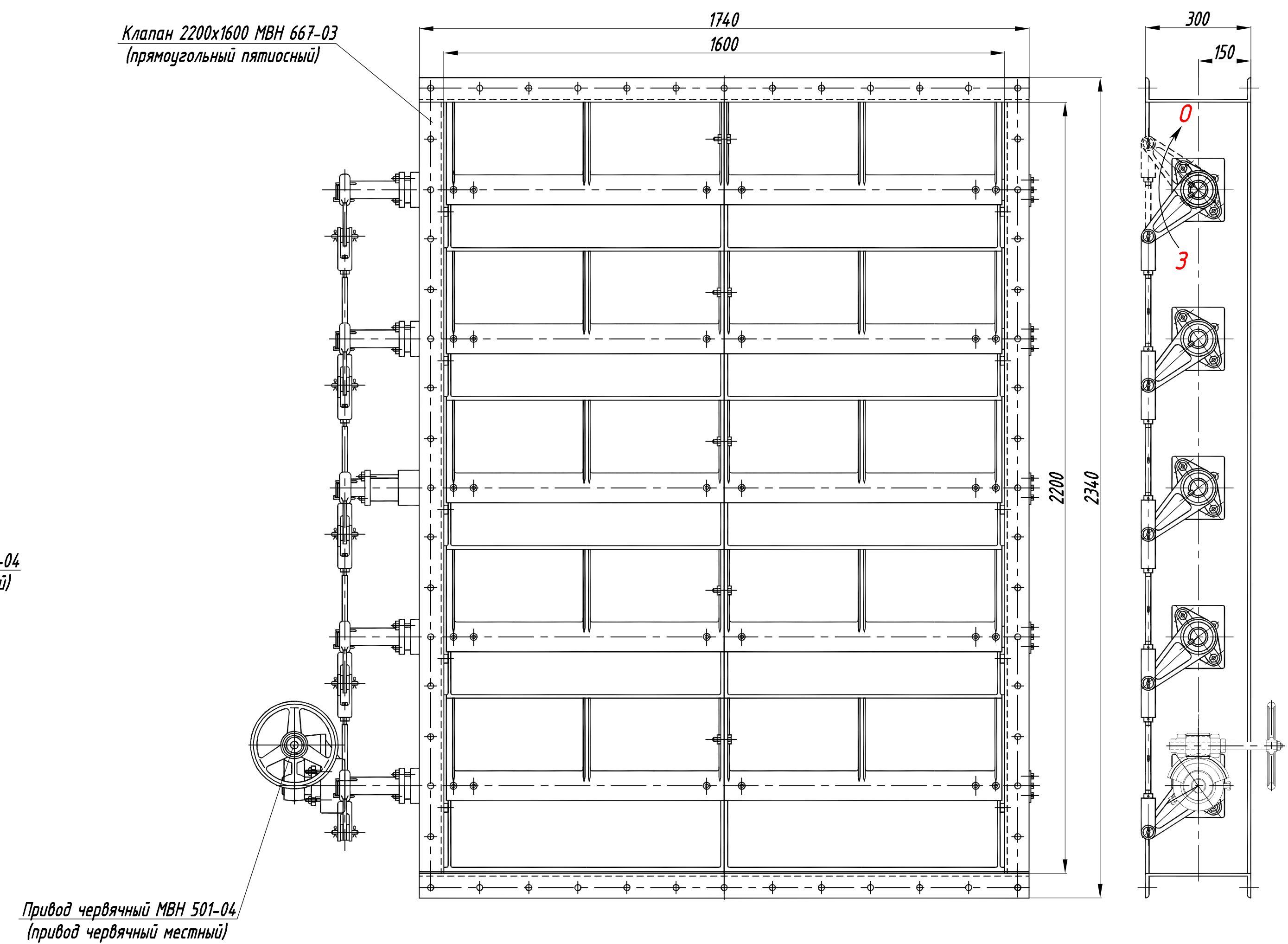
Клапан с левым расположением местного привода.
