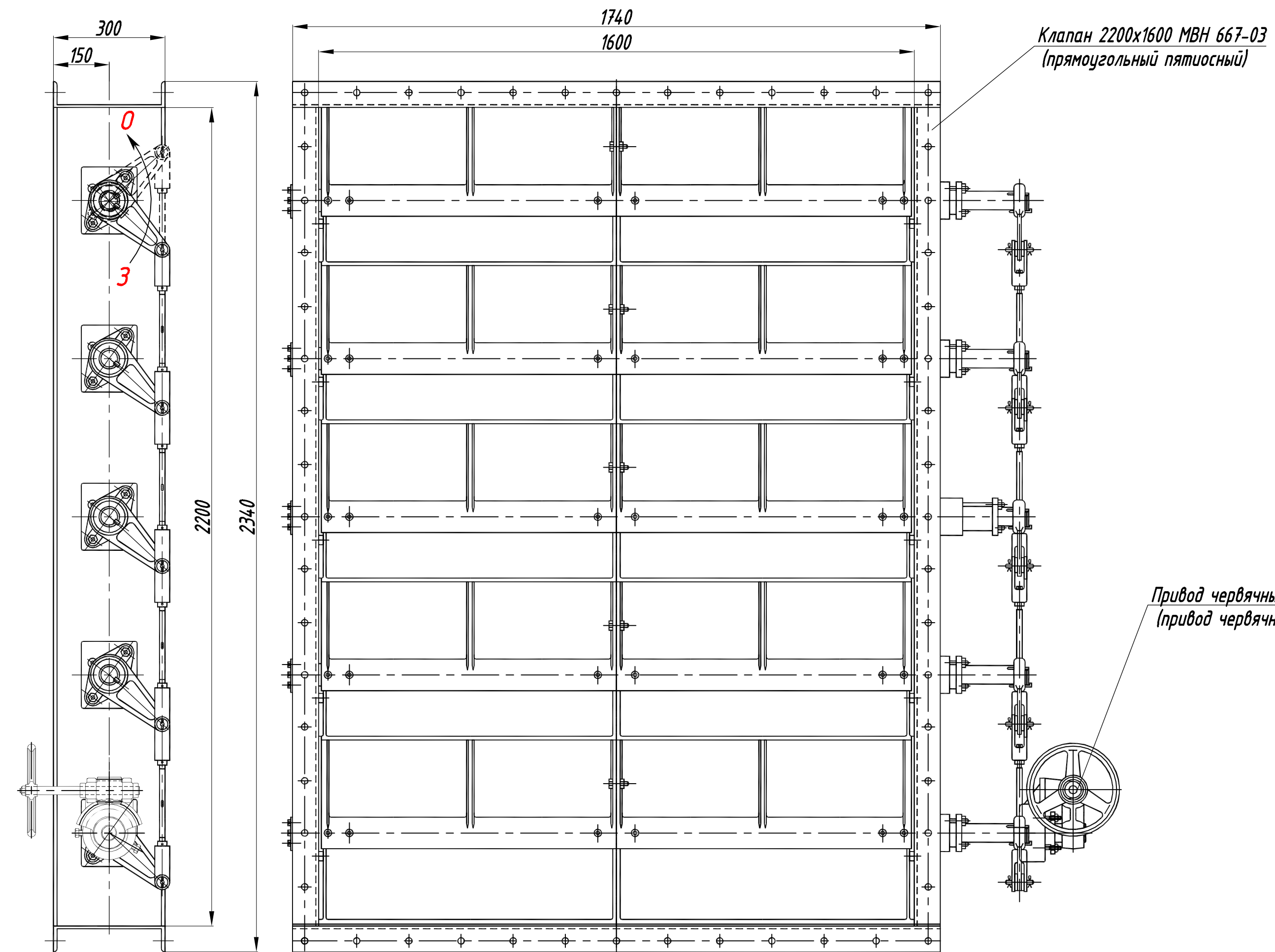
Клапан с правым расположением местного привода.
