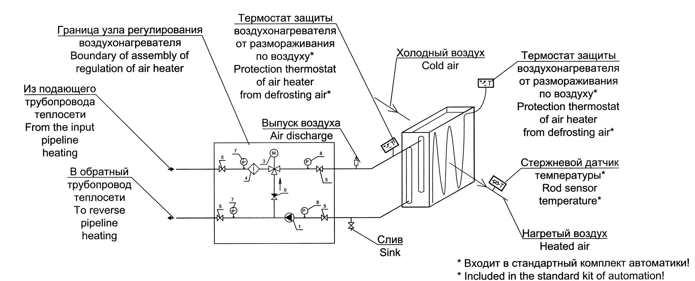
Принципиальная схема узла регулирования воздухоподогревателя систем 30SAH42 AH001 - 30SAH42 AH057 Schematic diagram of the assembly of regulation of air heater of systems 30SAH42 AH001 - 30SAH42 AH057
