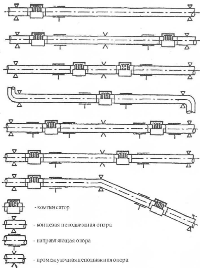
Рисунок 2. Схемы размещения компенсаторов и опор на трубопроводах
